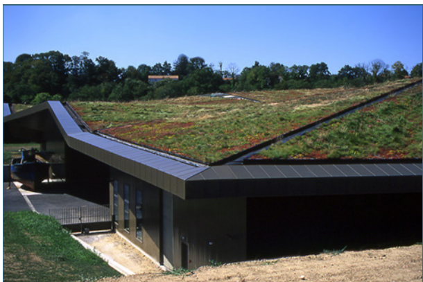
Abb. 4: Mit einem Gründach lassen sich bis zu 70 Prozent des anfallenden Niederschlags zurückhalten.
