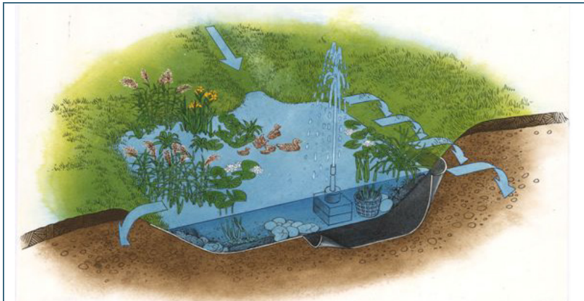
Abb. 6: Abfließendes Wasser kann auch in einen Sickerteich geleitet werden. Im Beispiel versickert das Wasser nicht am Grund, sondern an den oberen Rändern des Teichs. Der Sickerteich kombiniert Versickerung und Rückhaltung.
