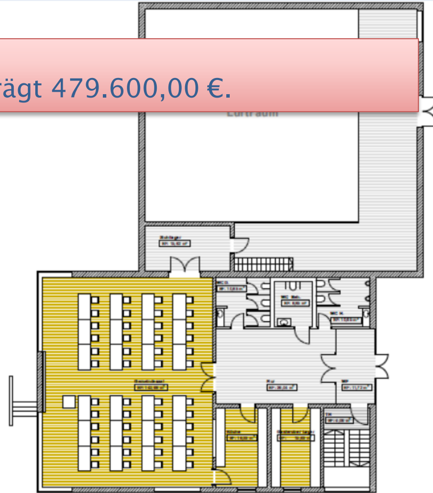
1. Obergeschoss
